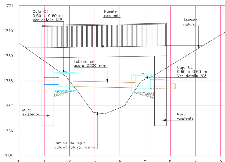
Esquema perfil transversal de la obra propuesta.
